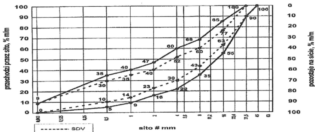
Rysunek 3. Uziarnienie mieszanki niezwiązanej 0/31,5 do podbudowy zasadniczej
